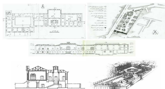
تصاویر ۱۴ تا ۱۸. پلان‌ها، سایت پلان و پرسپکتیو و مقطع عمارت مسعودیه، تهران؛ ماخذ: گزارش ثبتی عمارت مسعودیه، ۱۳۷۷
