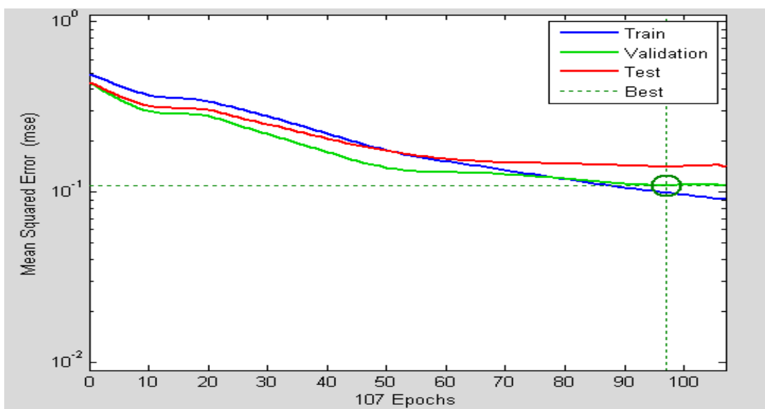
شکل (۵) کارایی مدل به ازای داده‌های آموزش، اعتبارسنجی و تست نمایش برای معماری ۱۵-۳۲-۱ (منبع: یافته‌های تحقیق)
