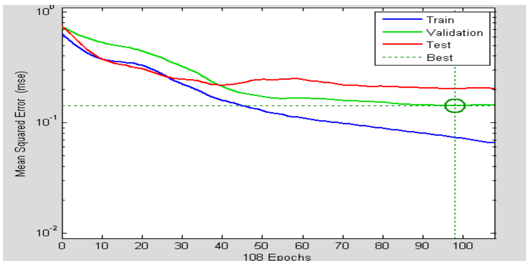
شکل (۴) کارایی مدل به ازای داده‌های آموزش، اعتبارسنجی و تست نمایش برای معماری ۱۵-۳۱-۱ (منبع: یافته‌های تحقیق)
