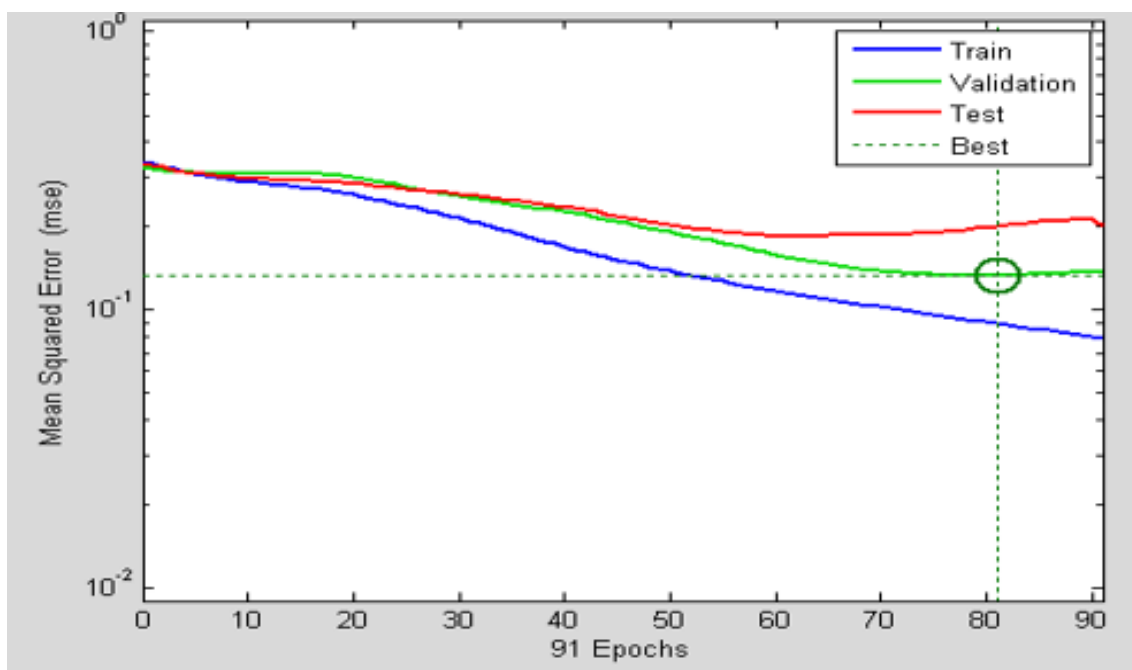
شکل (۱) کارایی مدل به ازای داده‌های آموزش، اعتبارسنجی و تست نمایش برای معماری ۱۵-۲۸-۱ (منبع: یافته‌های تحقیق)
