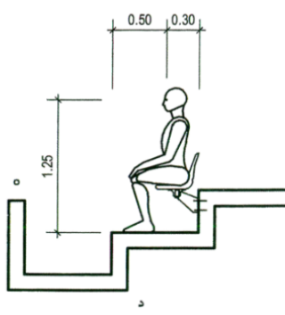
شکل ۲۱. حالات نشستن و ارتفاع دید
