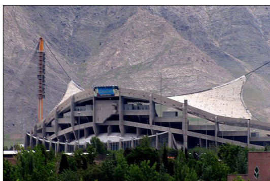
شکل ۳. استادیوم تختی تهران و سازه کابلی منحصراً بفرش؛ ماخذ: آرشیو نگارنده.
