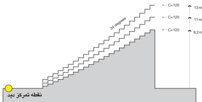
شکل ۱۴. محدوده آزاد دید
