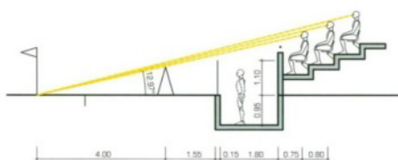
شکل ۱۱. نمونه ای از ابعاد استاندارد سکوهای تماشاچیان
