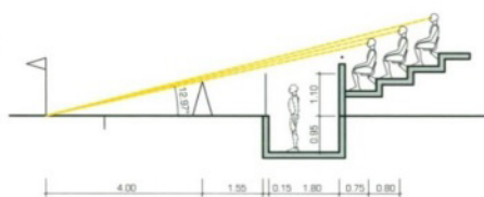
شکل ۱۱. نمونه ای از ابعاد استاندارد سکوهای تماشاچیان
