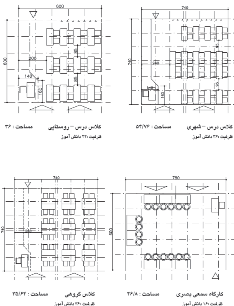
تصویر ۴. چیدمان کلاسهای مراکز آموزشی ابتدایی؛ مآخذ: ضوابط و استانداردهای سازمان نوسازی مدارس، ۱۳۹۱.
