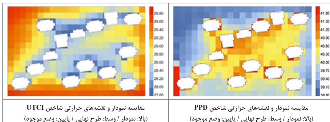
(شکل ۶) - مقایسه نمودار و نقشه‌های حرارتی شاخص‌های PET و PMV و PPD و UCI
