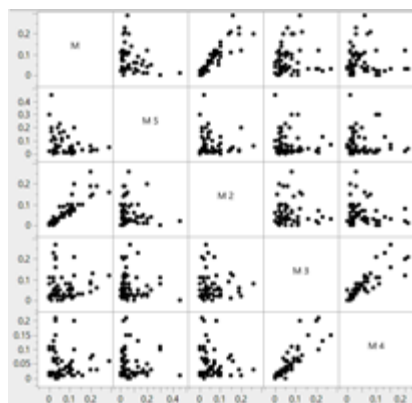
تصویر ۸: نمودار ماتریس همبستگی عوامل
