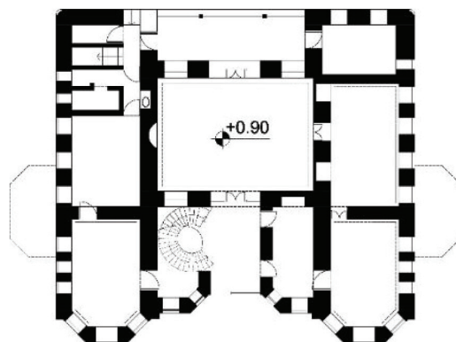
پلان طبقه اول
