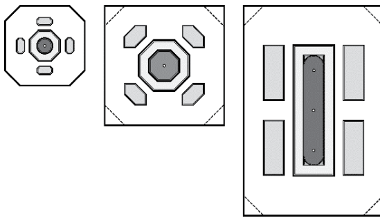
نمودار ۵. اشکال غالب و تناسبات تقریبی حیاط در خانه‌های سنتی عصر قاجار (از راست به چپ: اندرونی، بیرونی و نارنجستانی)؛ مأخذ: نگارنده
