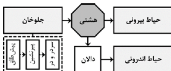
نمودار ۱. سلسله مراتب غالب ورودی در خانه‌های سنتی عصر قاجار؛ مأخذ: نگارنده
