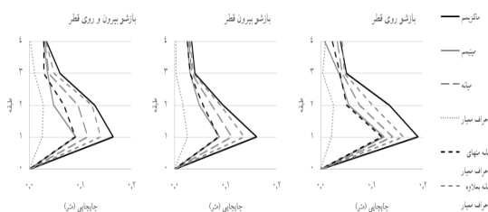
شکل ۱۰. میزان تغییر مکان ماکزیمم طبقات مختلف قاب با سیستم دیوار برشی فولادی با سه چیدمان مختلف بازشوهای چندگانه
