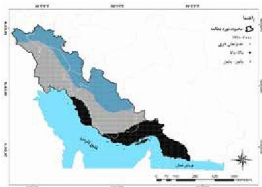
شکل ۱۴. پراکندگی فضایی نقاط بالا-بالا و پایین-پایین فشار بخار آب در دهه ۱۹۹۰-۲۰۰۰ در جنوب و جنوب غرب ایران
