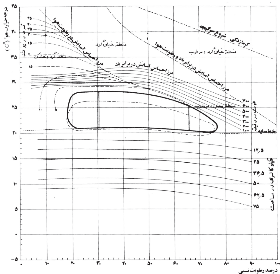
نمودار ۲. نمودار بیوکلیماتیک؛ ماخذ: کسمایی، ۱۳۶۳، ص ۱۷۳.
