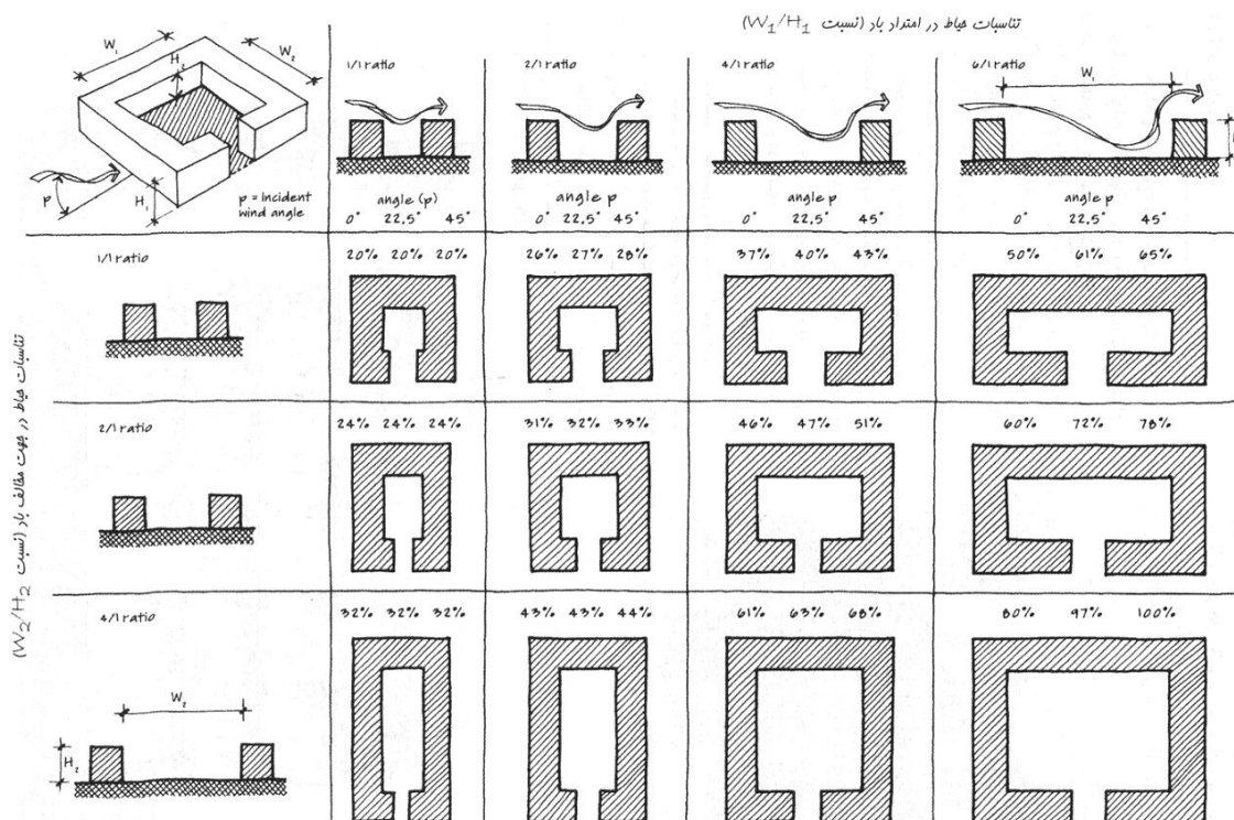
نمودار ۳. تعیین اندازه حیاط ابرای تهویه طبیعی؛ مأخذ: براون، ۱۳۸۶، ص ۲۰۹.
