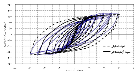
شکل ۴. مقایسه منحنی پسماند نمونه آزمایشگاهی وین و برونو و نمونه تحلیلی
