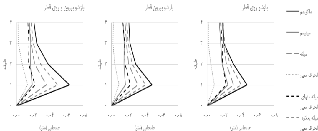
شکل ۹. میزان پراکنده‌گی پاسخ طبقات مختلف قاب با سیستم دیوار برشی فولادی با سه چیدمان مختلف بازشوهای چندگانه
